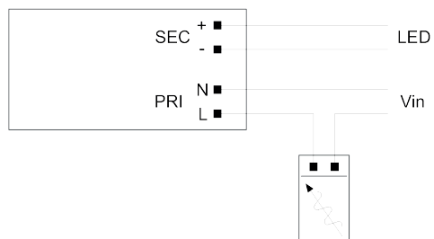
Schema di collegamento dimmerabile (IGBT - TRIAC) Dimmerable wirign diagram (TRAILING EDGE - LEADINJG EDGE)
